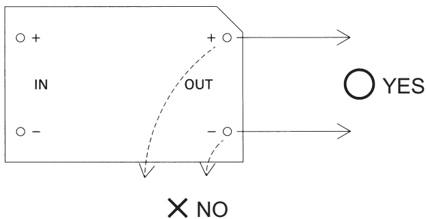
Fig.5.1 Pattern wiring
